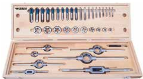
Gevindskæresæt UNF 1/4"-3/4" i trækasse.
